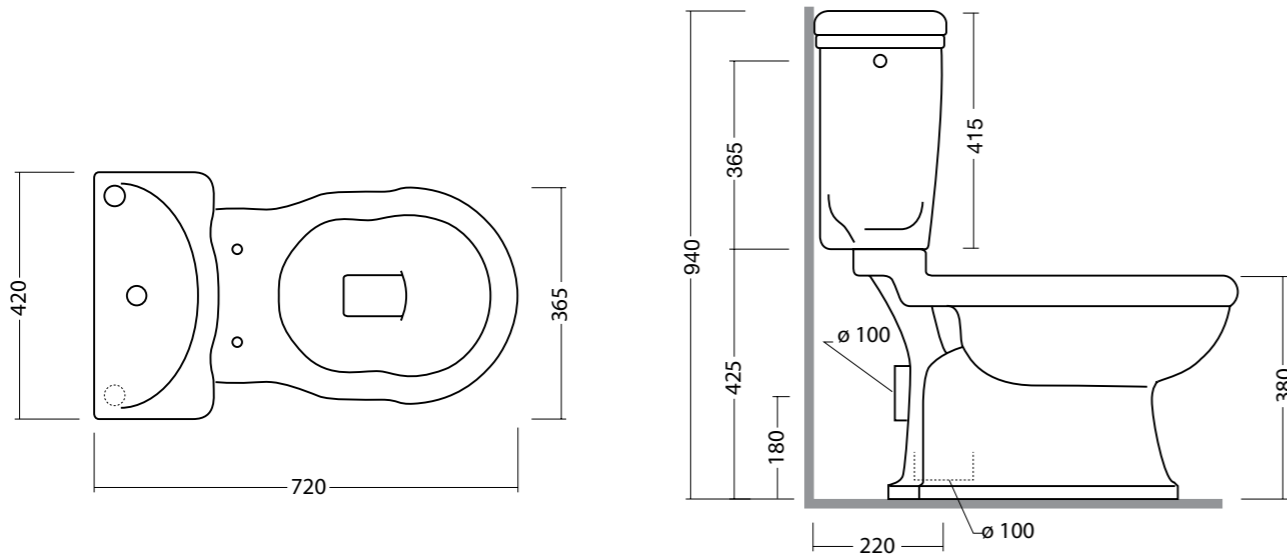
BOHEME vaso monoblocco cod. 28280101 Vaso boheme monoblocco con scarico a terra. Monobloc WC boheme with s outlet.
