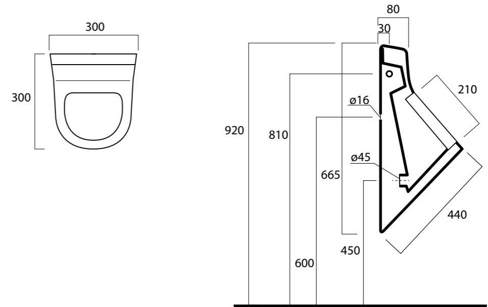
FORM orinatoio cod. 22260101 Orinatoio sospeso. Wall hung urinal.
