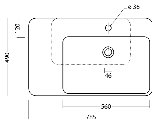
EDGE 80x50 cod. 26160101 Lavabo edge 80x50 monoforo. Installazione sospesa o ad appoggio. Washbasin edge 80x50 thin single tap hole. Wall hung or countertop installation.
